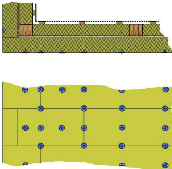
Obr. 5: Kladení fasádních tepelně izolačních desek na deskový podklad
