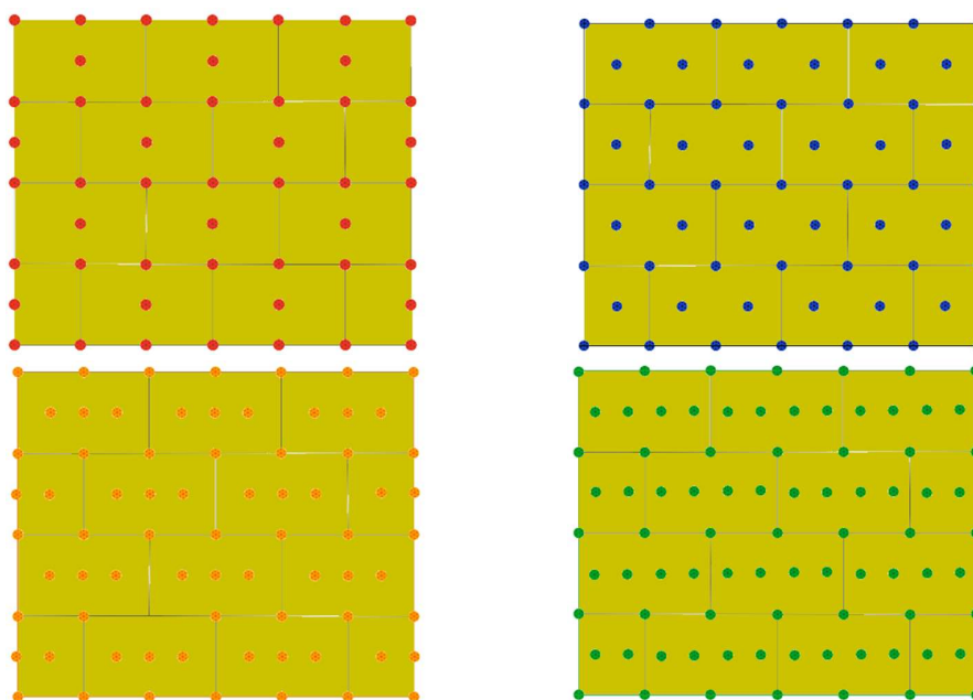
Obr. 8: Doporučený kotevní plán na desky 600×1000 mm
