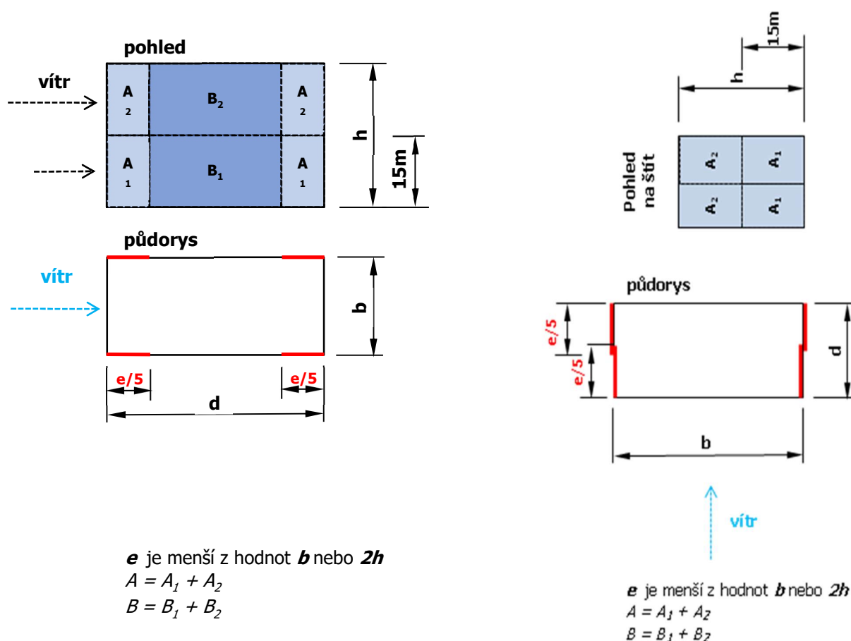
Obr. 10: Grafické znázornění jednotlivých parametrů pro stanovení okrajové a vnitřní oblasti plochy
