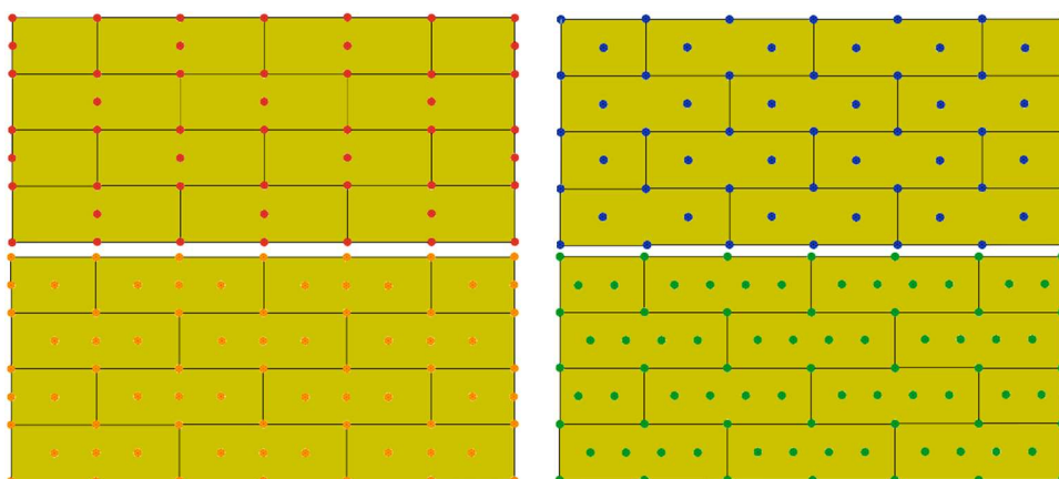
Obr. 9: Doporučený kotevní plán na desky 1 200×400 mm
