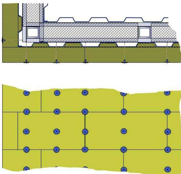
Obr. 6: Kladení fasádních tepelně izolačních desek na plechový podklad (nesmí vzniknout průběžná vertikální mezera větší jak 0,01 m 2 )
